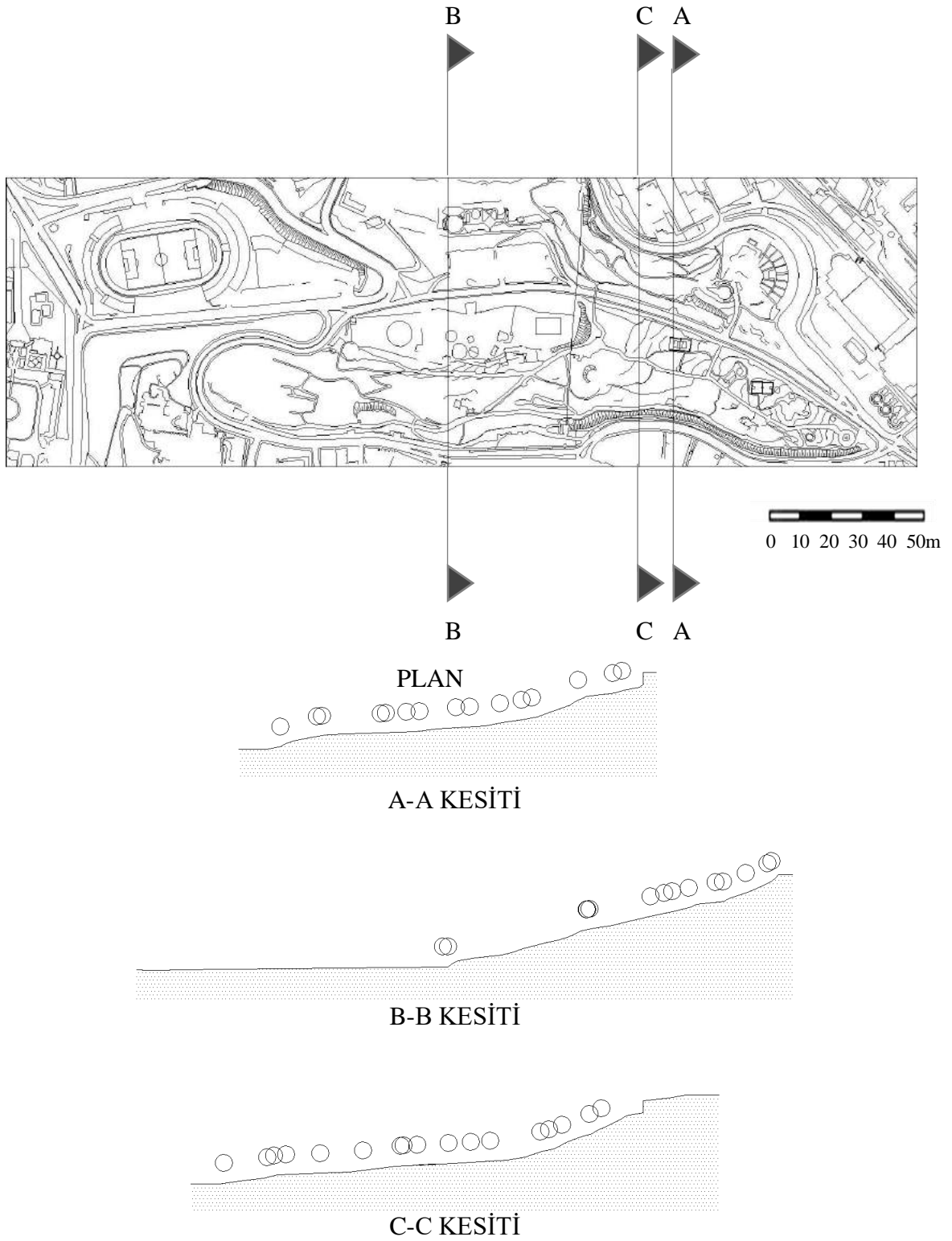
Şekil 2.6. Maçka Demokrasi Parkı Plan ve Kesitler
