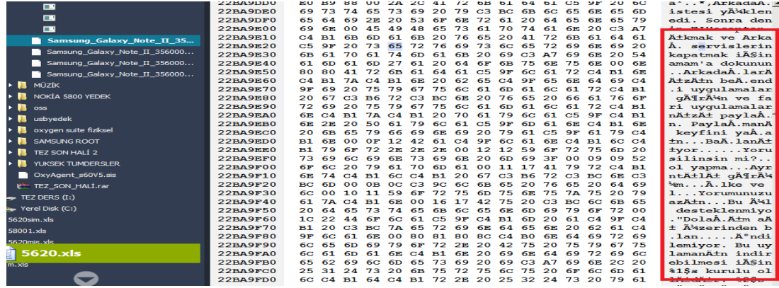
Şekil 49-Mobiledit ile tespit edilen Samsung GT-N7100 Web kaydı
