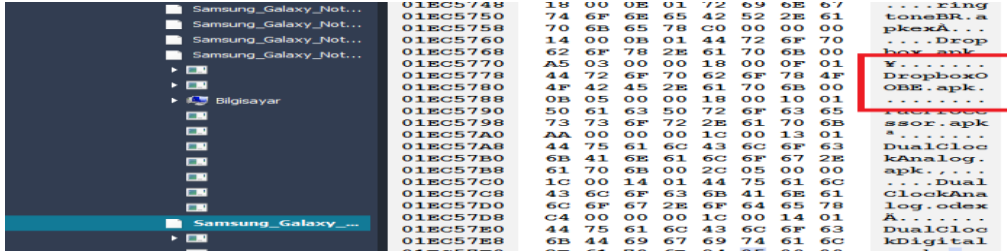
Şekil 53-Mobiledit ile tespit edilen Samsung GT-N7100 Uygulama Kaydı
