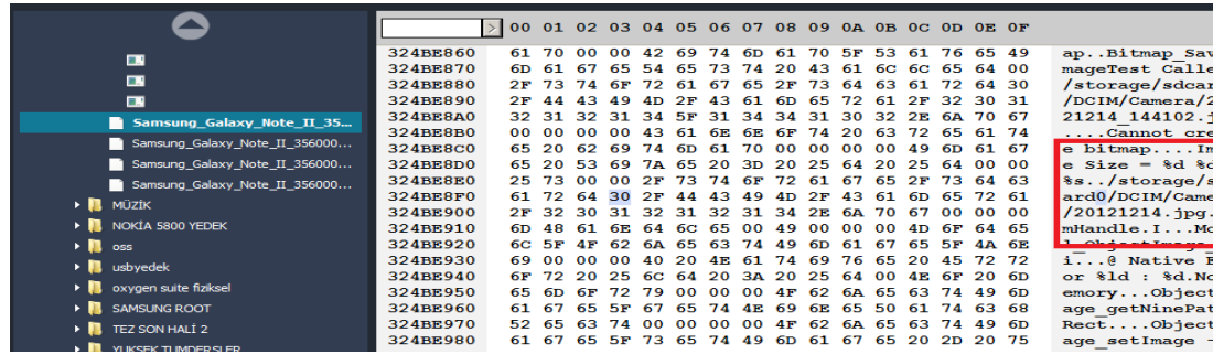
Şekil 50-Mobiledit ile tespit edilen Samsung GT-N7100 resim dosyası bilgisi.
