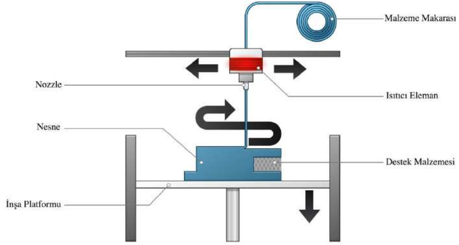
Şekil 4.2. Eklemeli Üretim Yöntemi (FDM. Çev. Yazar) (Url-10).
