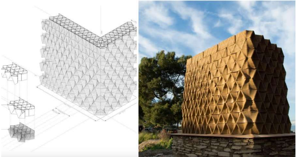
Şekil 5.2. TerraPerforma Dijital Tasarım ve Üretim Yaklaşımları (Url-12).
